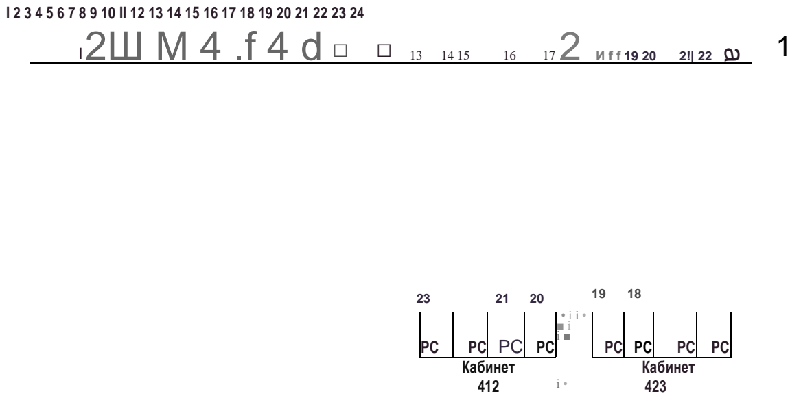
Коммутатор 2 (24 порта)
